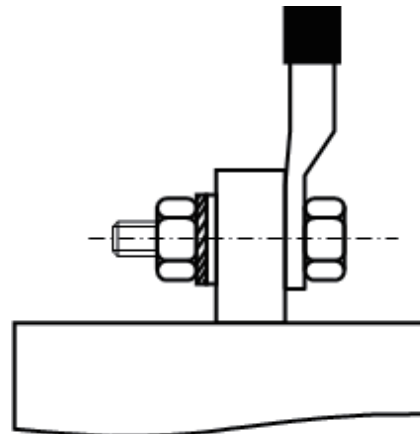
Abb 2: Anschluss an den Batteriepol mit Unterlegscheibe
